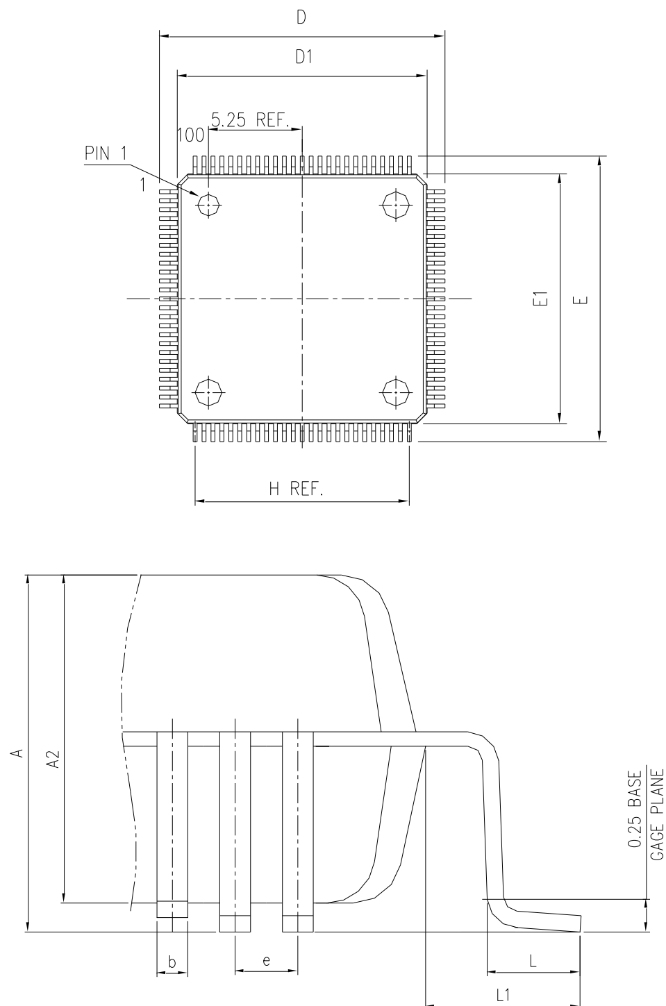
图 14 LQFP100 封装图
