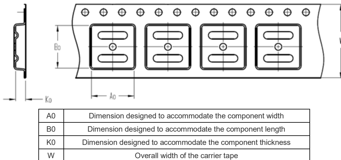
图 19 带状包装规格图
